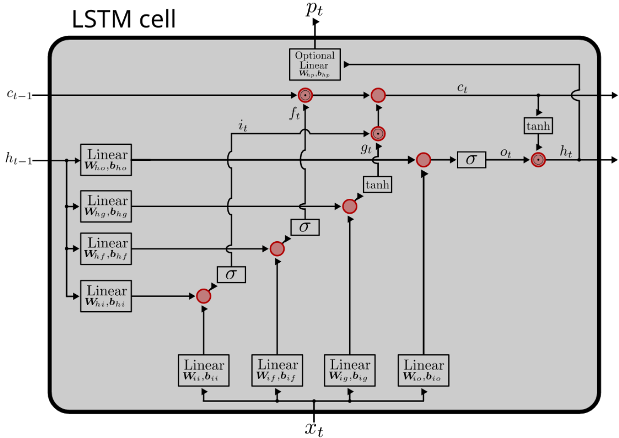
Rysunek 2.2. Schemat komórki LSTM. Źródło: [27].
